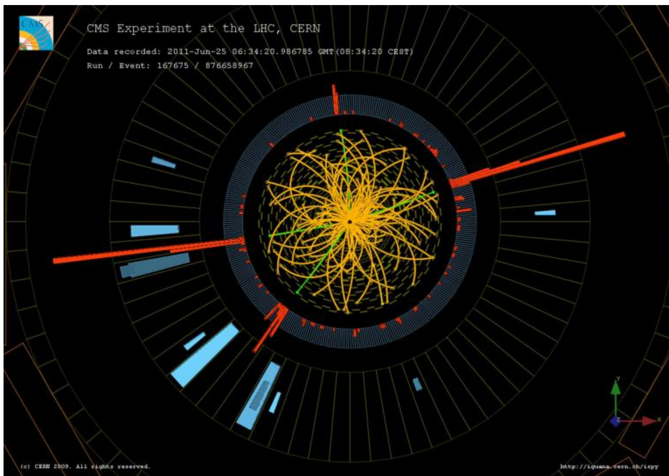
Il bosone di Higgs.
