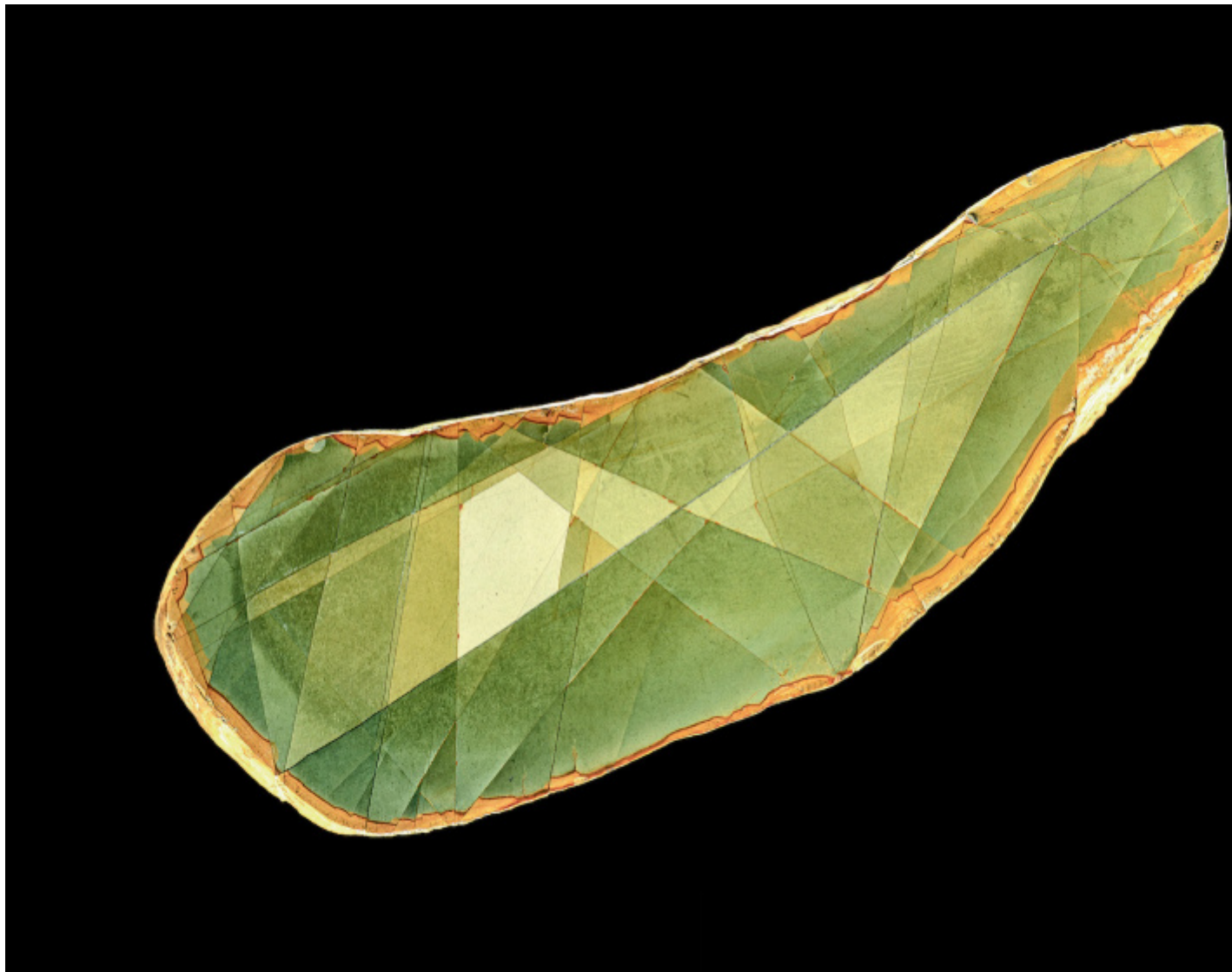
Calcare, varietà toscana detta Verde d'Arno Alta Valle dell'Arno (Firenze, Italia) blocco segato e levigato su un lato 15,1 x 5,9 cm Donazione Caillois, 1984-1985 MNH, INV. 188.94.
