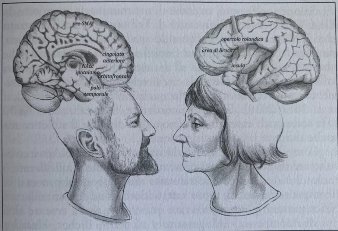
FIG. 6. Le neuroscienze della risata emozionale e volontaria. Visione mesiale (sinistra) e laterale (destra) del cervello. Per questa immagine, hanno prestato il proprio profilo (ma non il proprio cervello!) gli autori di questo libro.
